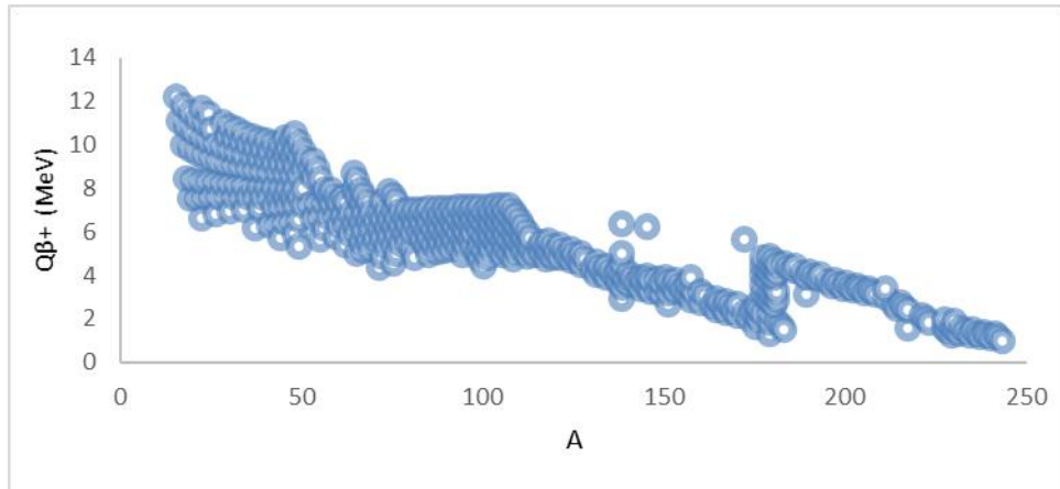
الشكل 7: العلاقة بين طاقة انحلال بيتا الموجبة ( Q_{\beta}^{+} ) والعدد الكتلي ( A )
